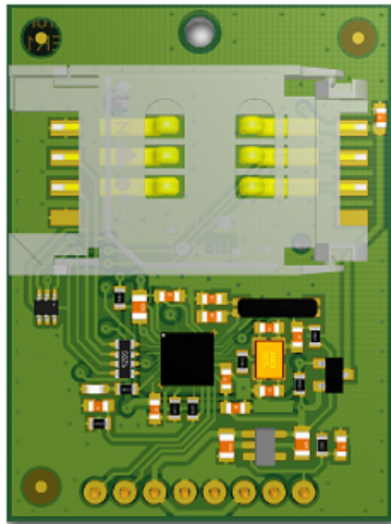
Top Side
